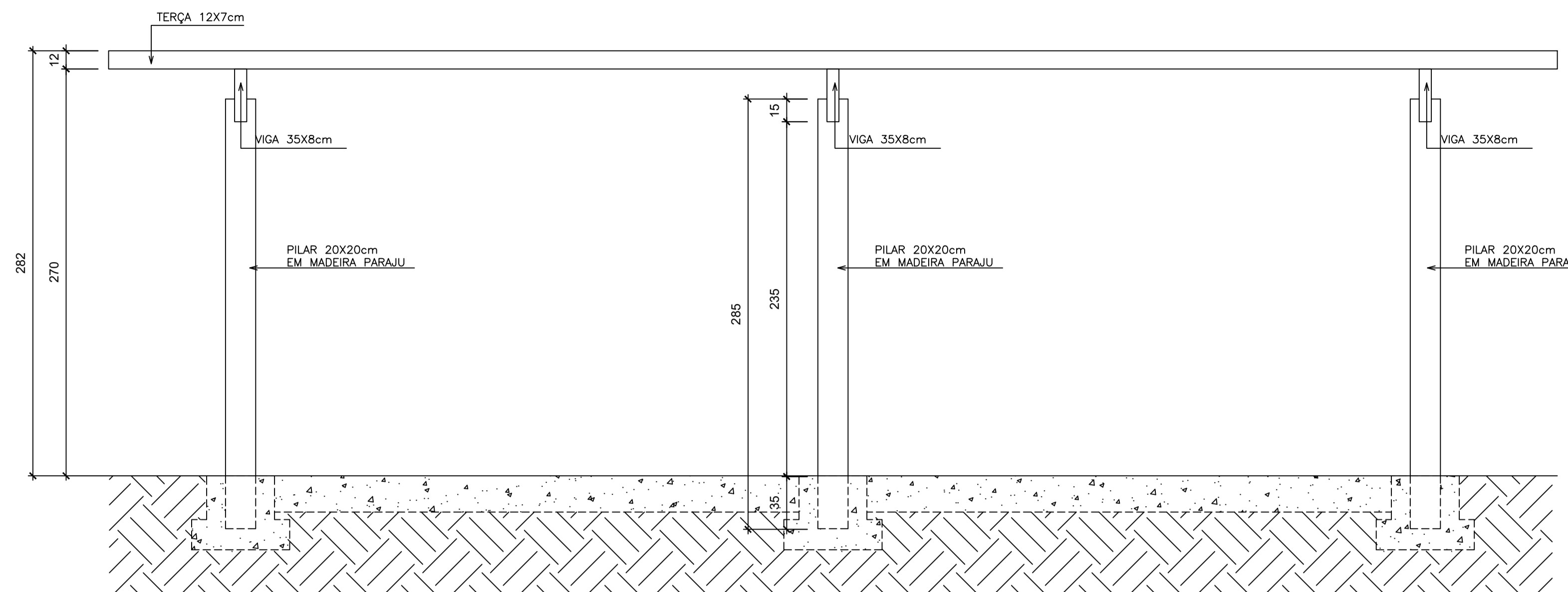
VISTA 2 PERGOLADO - PRAÇA SAUDAVÉL - MODELOS 1 E 2 ESCALA 1:25
