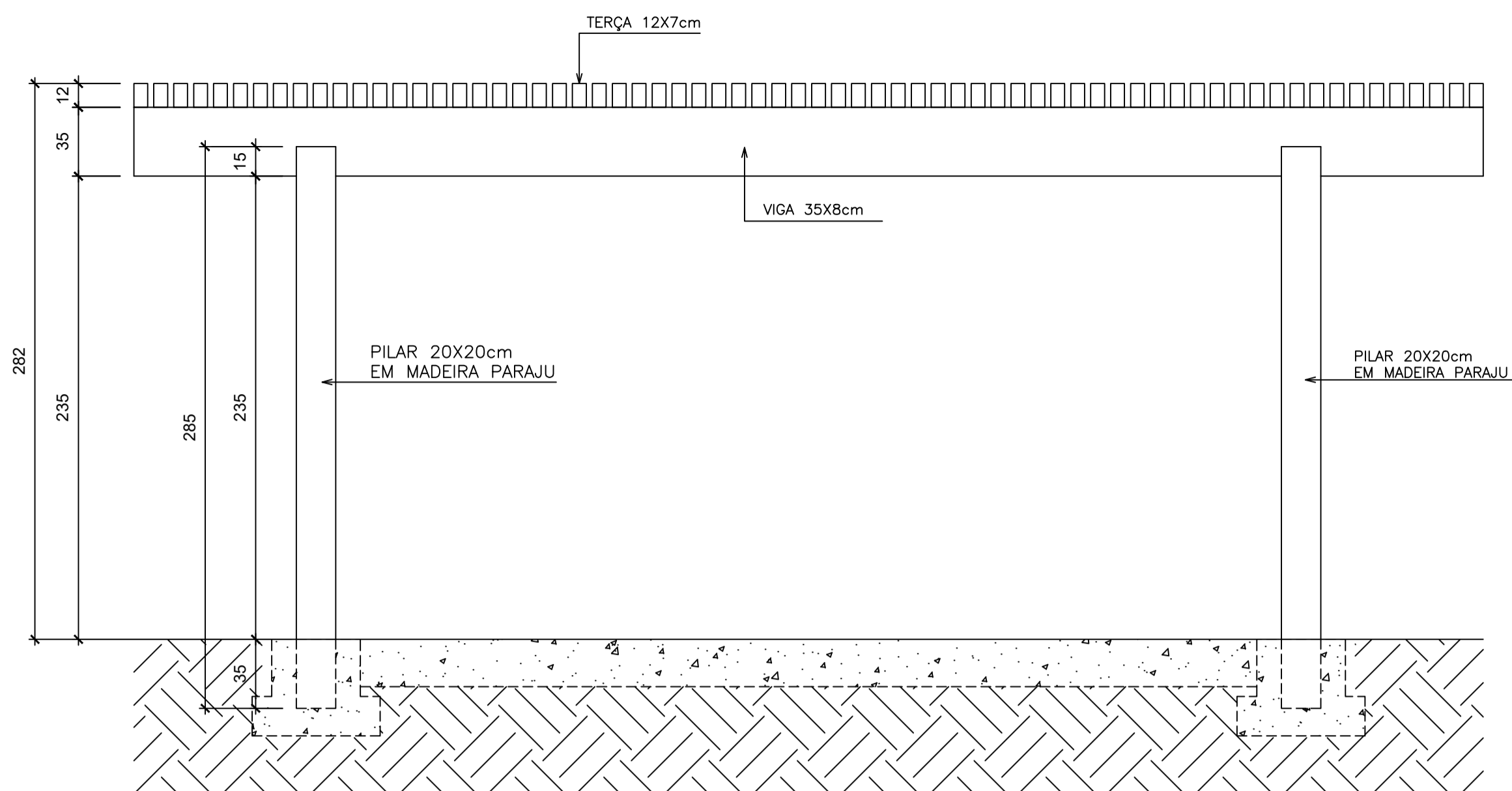
VISTA 1 PERGOLADO - PRAÇA SAUDAVÉL - MODELOS 1 E 2 ESCALA 1:25
