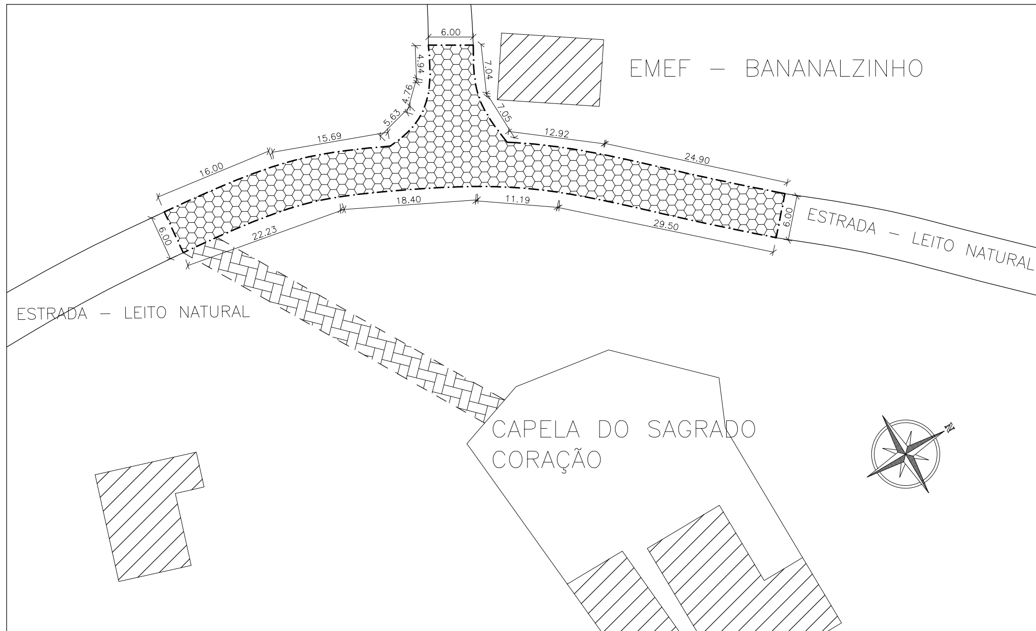
PLANTA BAIXA – PAVIMENTAÇÃO ESCALA 1:500
