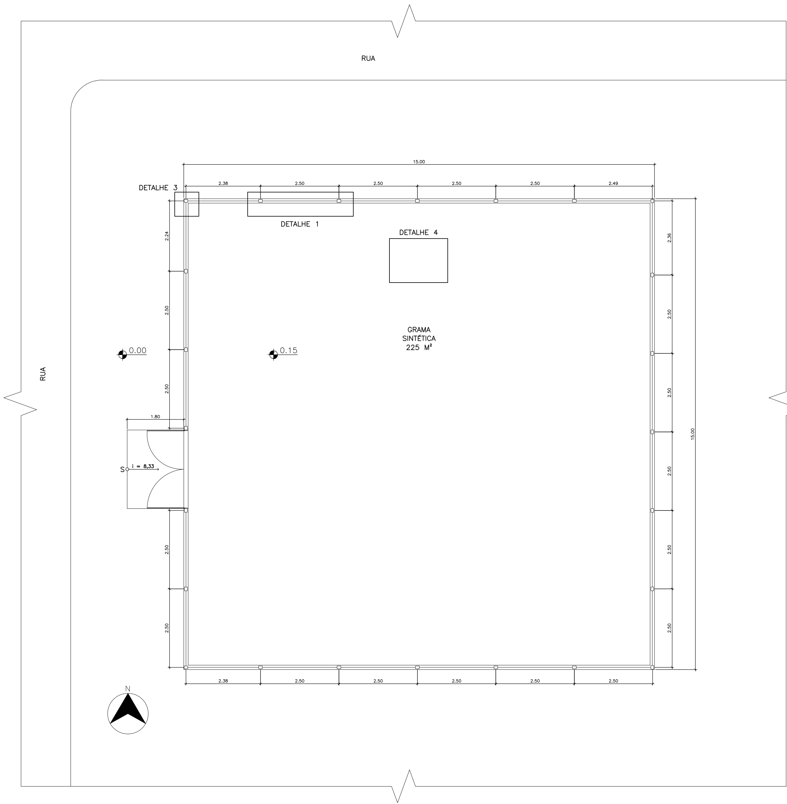
PLANTA BAIXA - LOCAÇÃO DO PARQUINHO INFANTIL ESC.: 1/50 COMPRIMENTO TOTAL DO CERCAMENTO COM PAINEL NYLOFOR 3D = 60 m
