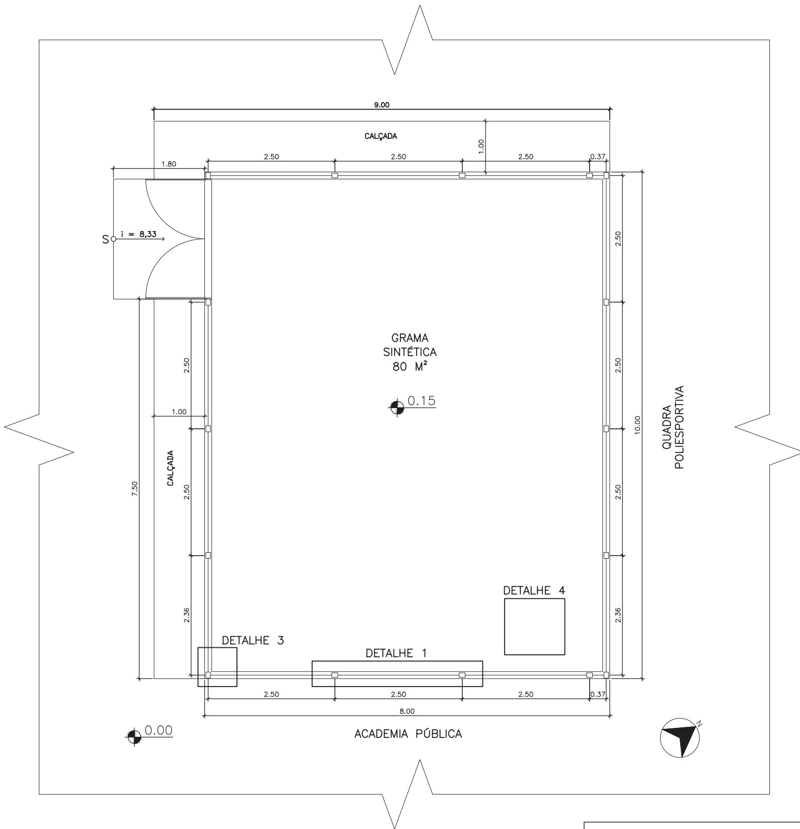
PLANTA BAIXA - LOCAÇÃO DO PARQUINHO INFANTIL ESC.: 1/50 COMPRIMENTO TOTAL DO CERCAMENTO COM PAINEL NYLOFOR 3D = 36 m
