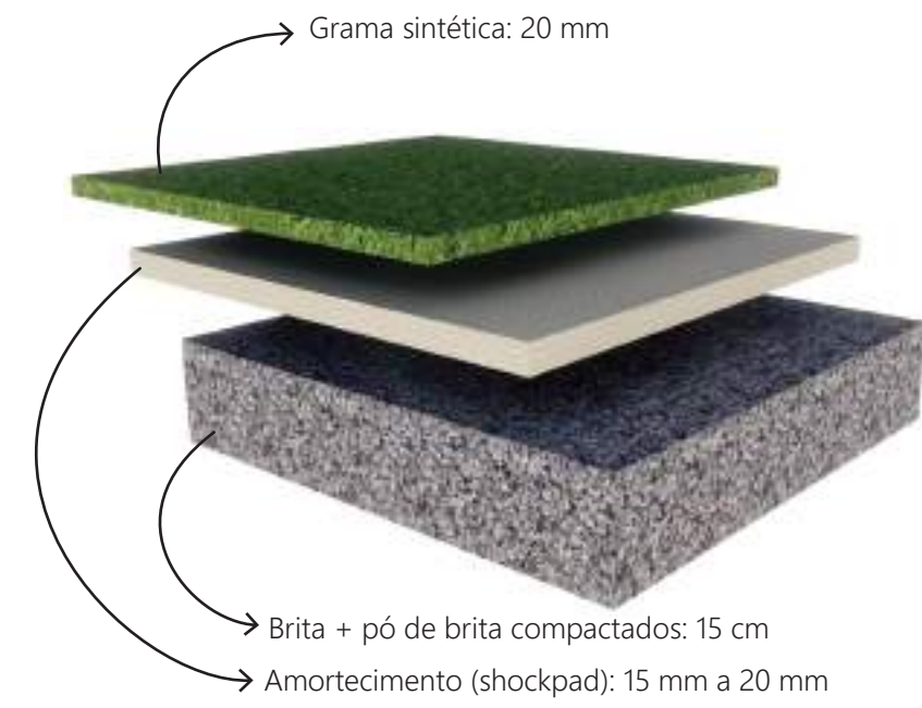
DETALHE 3 - ELEMENTOS DO GRAMADO
