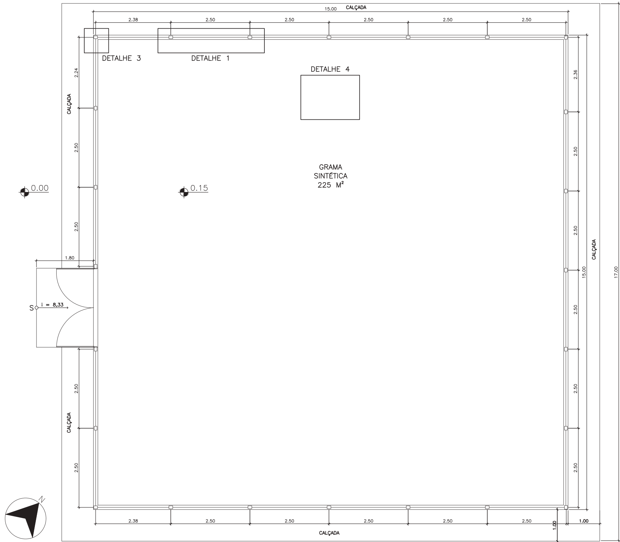
PLANTA BAIXA - LOCAÇÃO DO PARQUINHO INFANTIL ESC.: 1/150 COMPRIMENTO TOTAL DO CERCAMENTO COM PAINEL NYLOFOR 30 = 60 m
