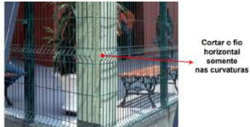
DETALHE 3 - CURVA DE PAINEL
