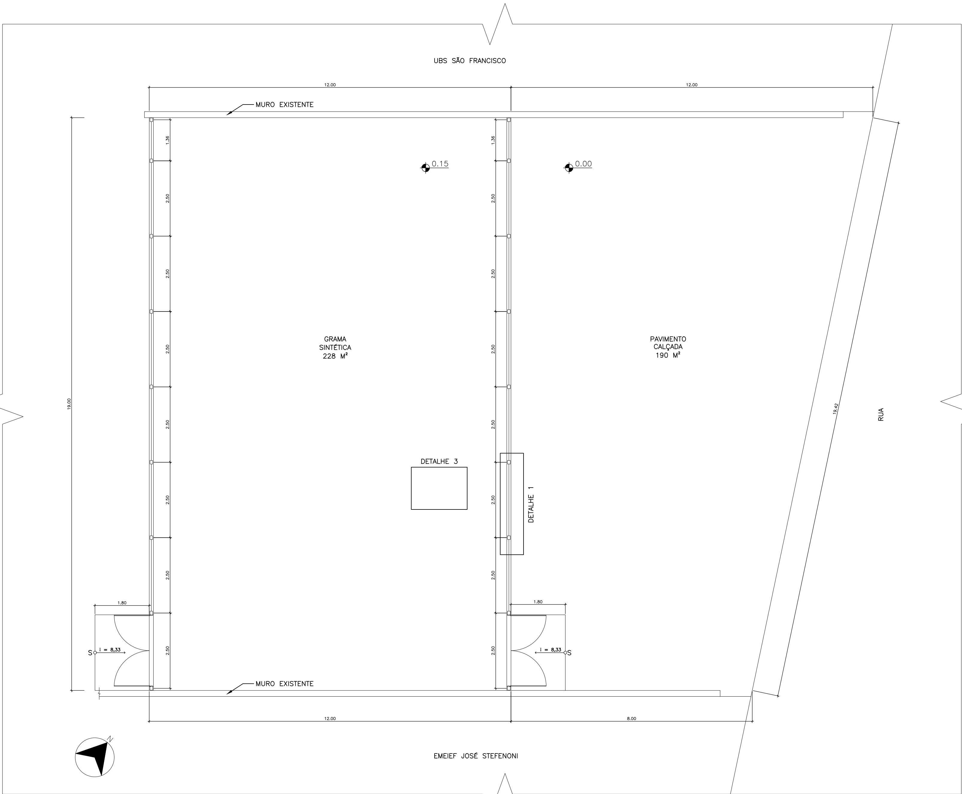
PLANTA BAIXA - LOCAÇÃO DO PARQUINHO INFANTIL ESC.: 1/50 COMPRIMENTO TOTAL DO CERCAMENTO COM PAINEL NYLOFOR 30 = 38 m
