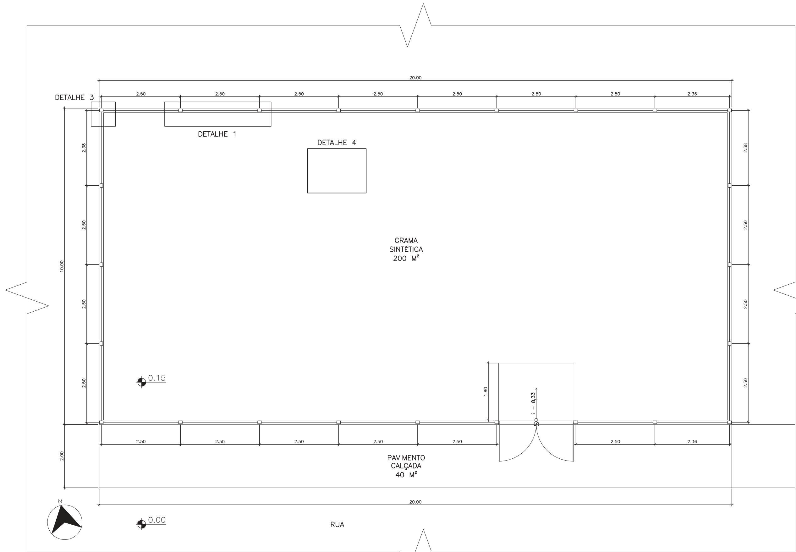
PLANTA BAIXA - LOCAÇÃO DO PARQUINHO INFANTIL ESC.: 1/50 COMPRIMENTO TOTAL DO CERCAMENTO COM PAINEL NYLOFOR 3D = 60 m
