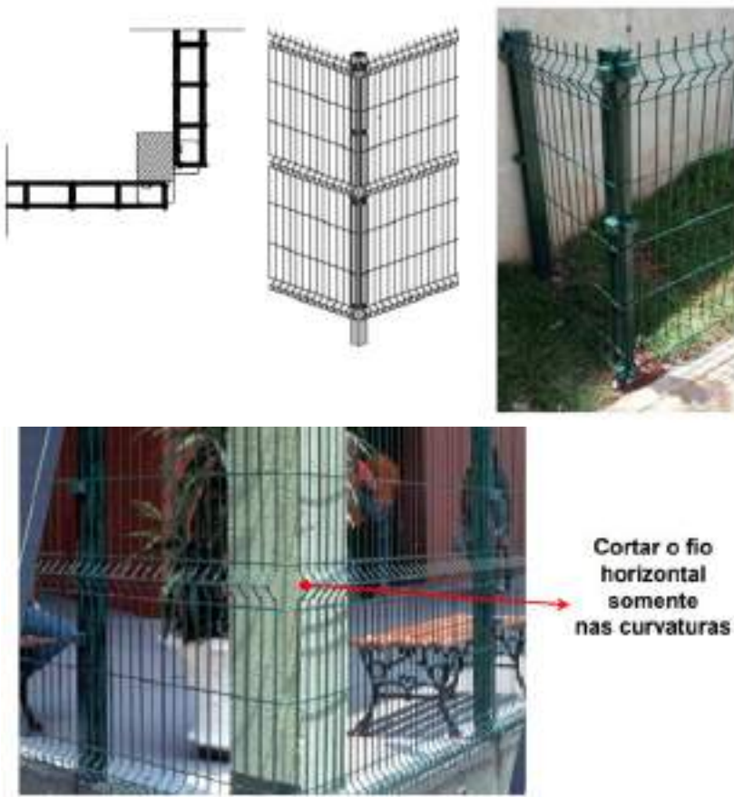
DETALHE 3 - CURVA DE PAINEL
