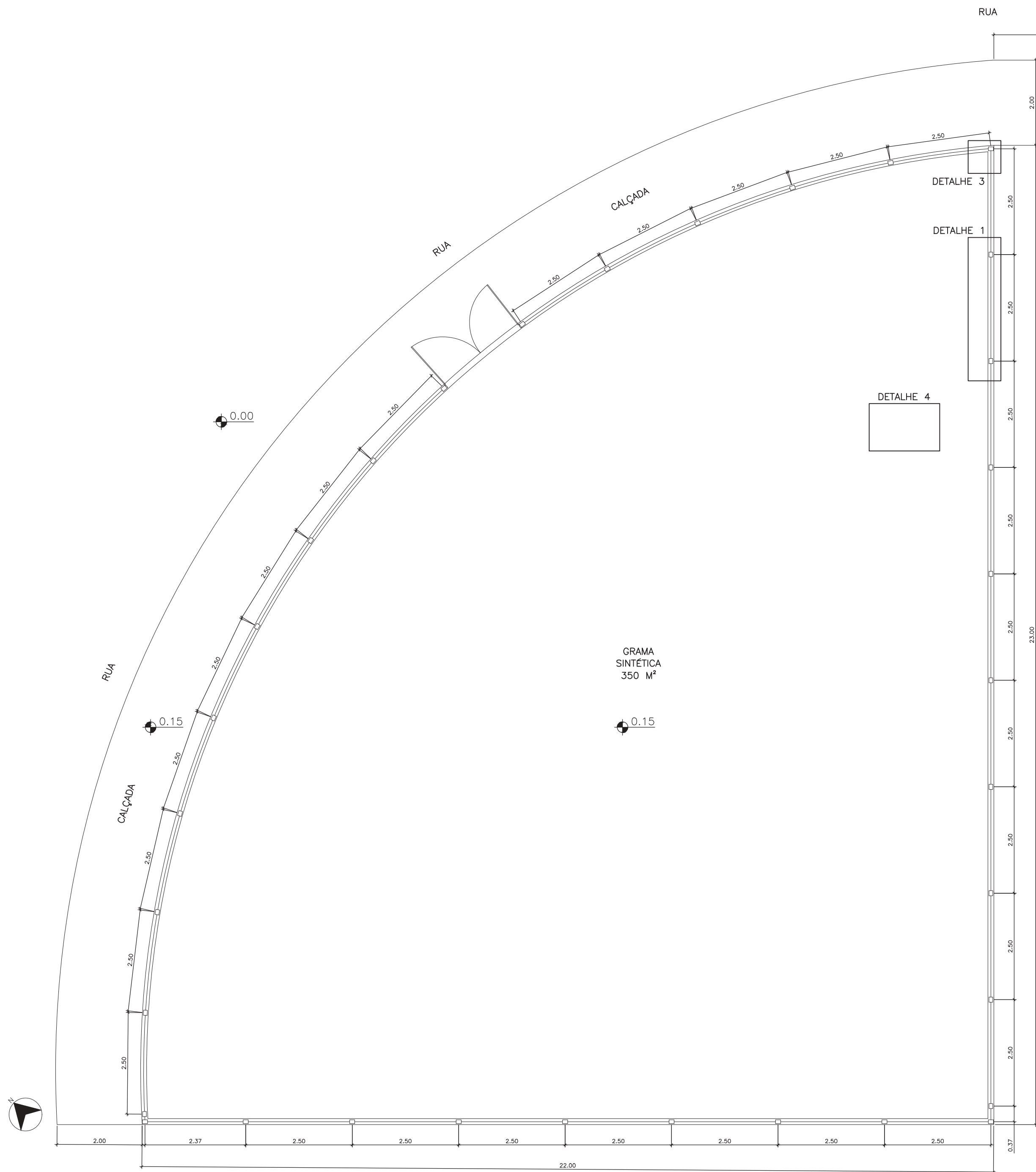
PLANTA BAIXA - LOCAÇÃO DO PARQUINHO INFANTIL ESC.: 1/50 COMPRIMENTO TOTAL DO CERCAMENTO COM PAINEL NYLOFOR 3D = 62 m
