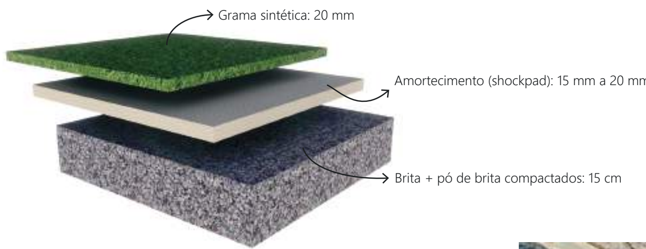
DETALHE 4 - ELEMENTOS DO GRAMADO
