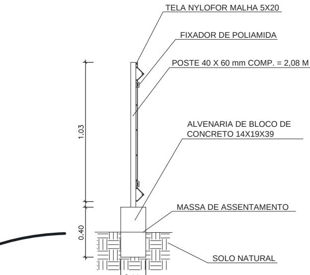
DETALHE 2 - SEÇÃO TRANSVERSAL ESC.: 1/20
