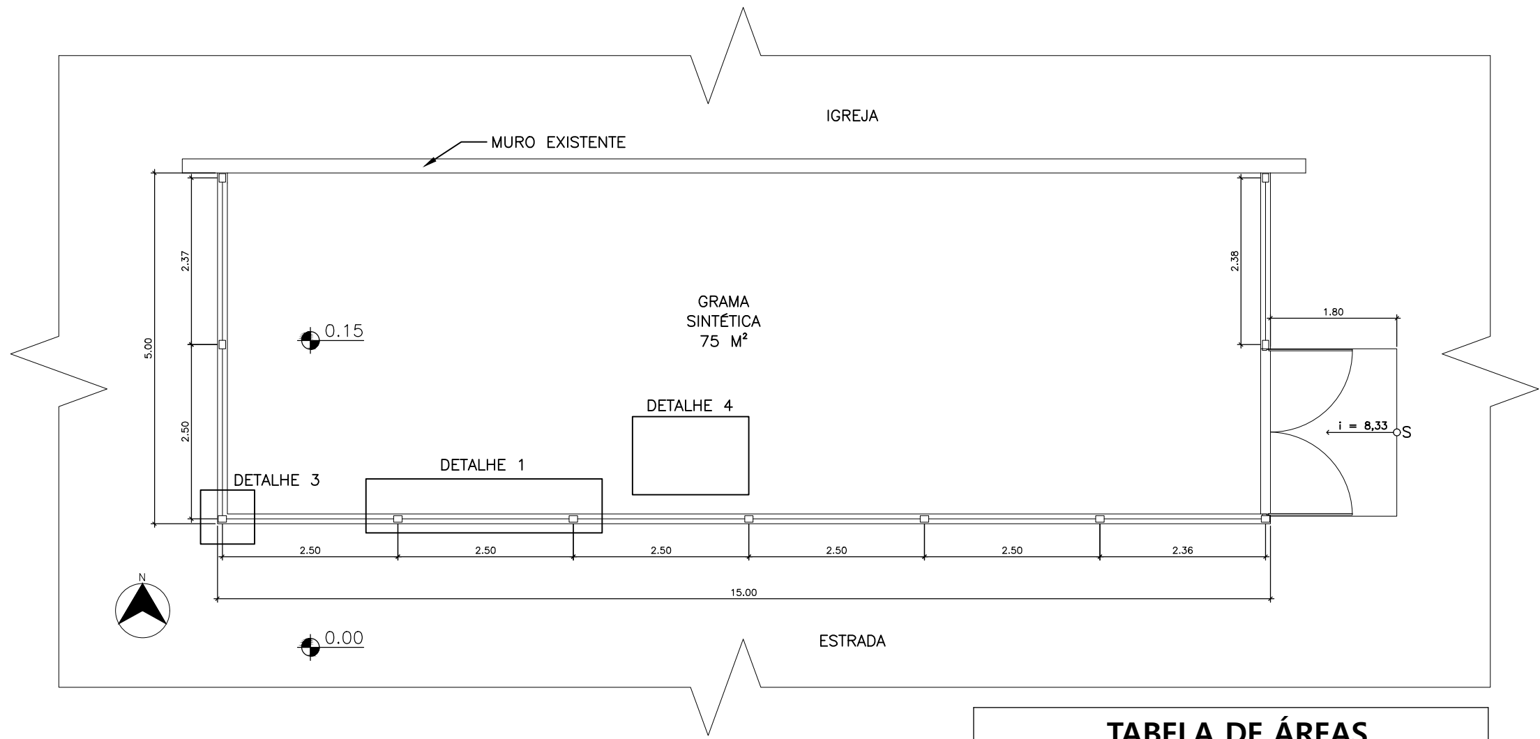
PLANTA BAIXA - LOCAÇÃO DO PARQUINHO INFANTIL ESC.: 1/50 COMPRIMENTO TOTAL DO CERCAMENTO COM PAINEL NYLOFOR 3D = 25 m
