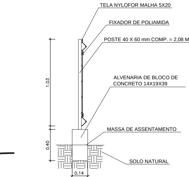
DETALHE 2 - SEÇÃO TRANSVERSAL ESC.: 1/20
