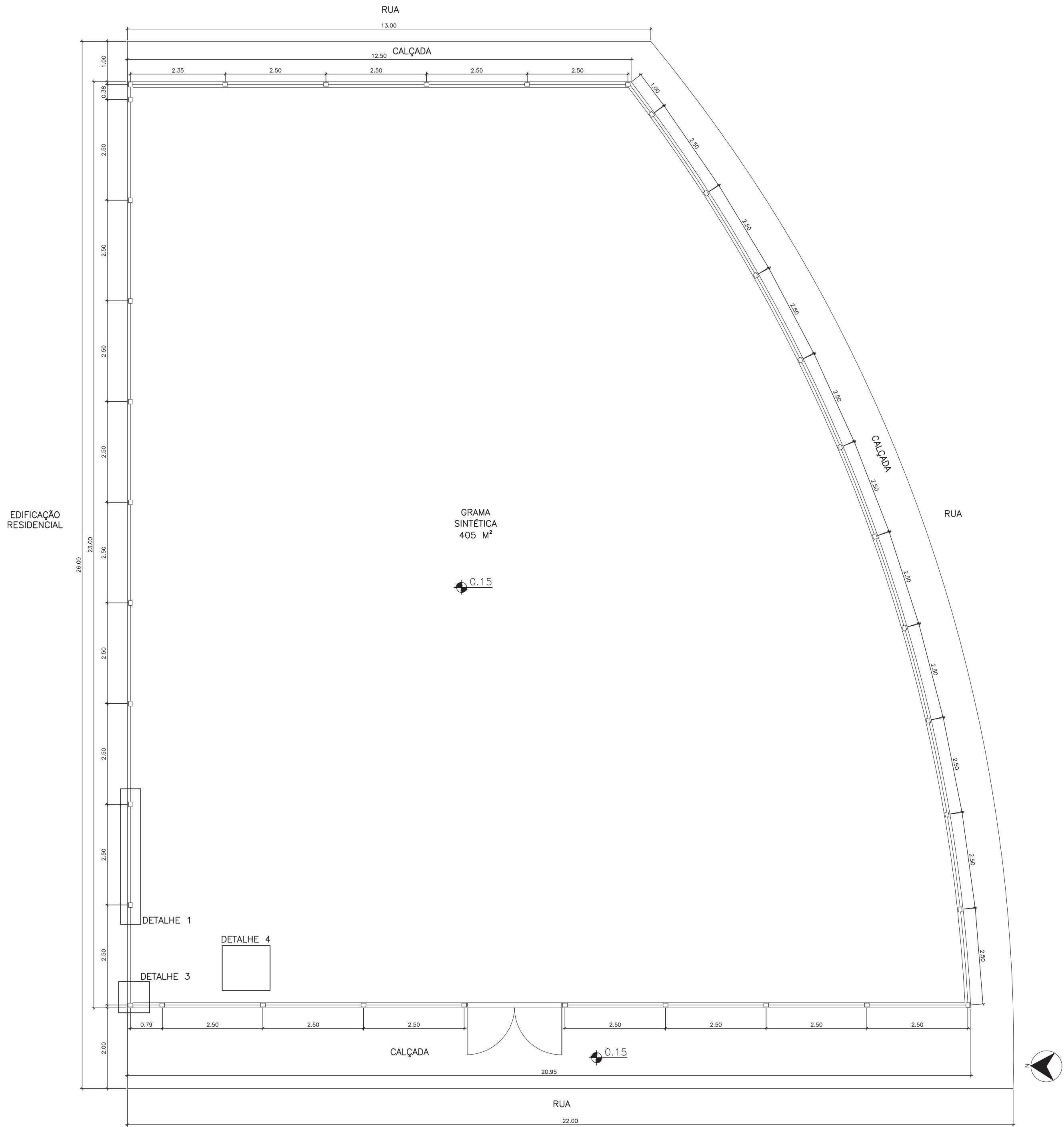
PLANTA BAIXA - LOCAÇÃO DO PARQUINHO INFANTIL
