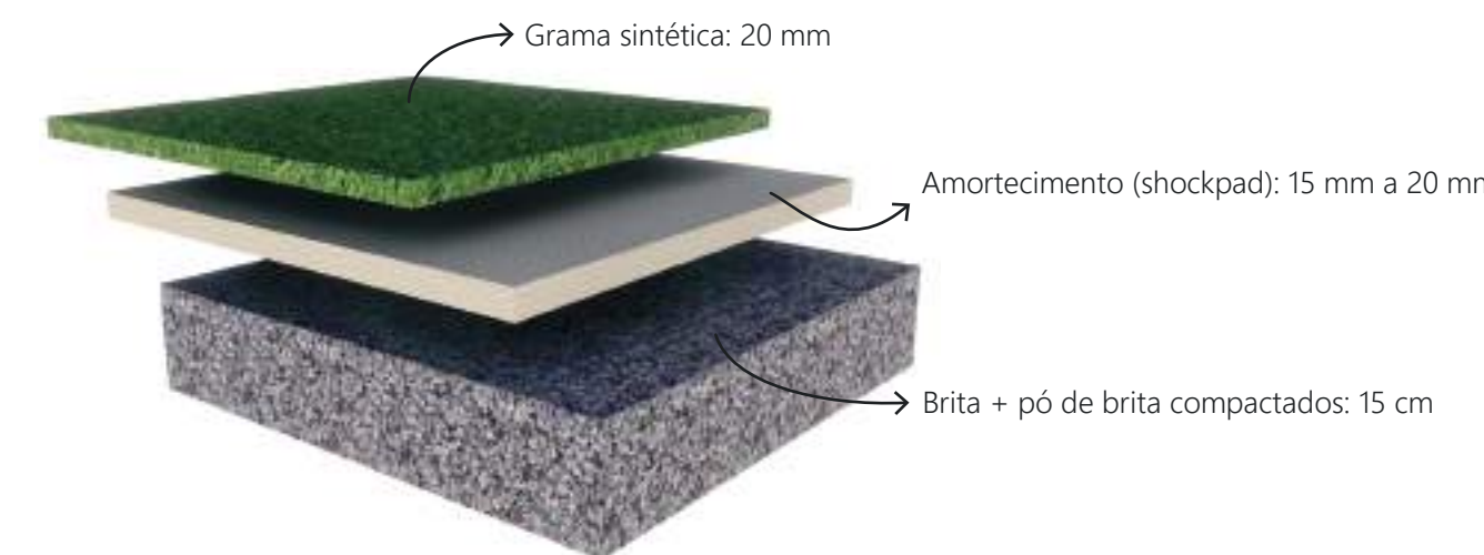
DETALHE 4 - ELEMENTOS DO GRAMADO
